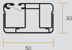
Coulisse télescopique (version motorisée) Telescopic guide (motorized version)
